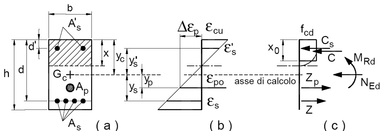
Figura 4.1.3– Sezione pressoinflessa
