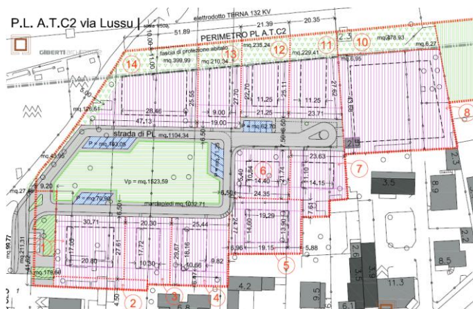
Planimetria dell'area
