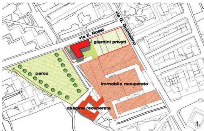
Schema planivolumetrico dell'area
